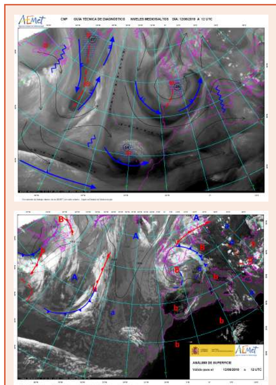
Figura A-A7 — Guía técnica de niveles altos y análisis de superficie del día 12 de junio a las 12 UTC. Fuente EUMETSAT/AEMET.
