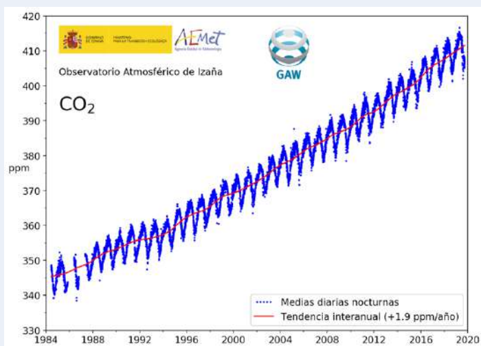
Figura 6 — Dióxido de carbono atmosférico (fracción molar diaria nocturna media) medido en el Observatorio de Izaña desde 1984, y tendencia interanual calculada a partir de esos datos. Superpuesta a la creciente tendencia interanual (debida a las emisiones antropogénicas), hay un ciclo estacional (crecimiento neto de biomasa durante la primavera y el verano del hemisferio norte, que implica una disminución del dióxido de carbono atmosférico; disminución neta de biomasa durante el otoño y el invierno del hemisferio norte, que implica un aumento del dióxido de carbono atmosférico). Fuente AEMET.
