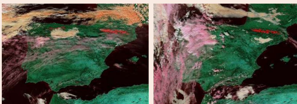
Figura A-A15 — Imagen MODIS del satélite SUOMI-NPP del 24 y 25 a mediodía. Fuente https://worldview.earthdata.nasa.gov .
