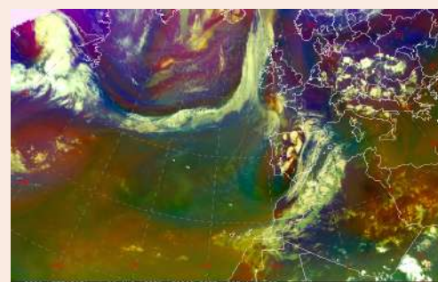
Figura A-A9 — Imágenes del satélite METEOSAT de las 15 UTC del día 26: vapor de agua (arriba) y masas de aire (abajo). Fuente https://worldview.earthdata.nasa.gov .
