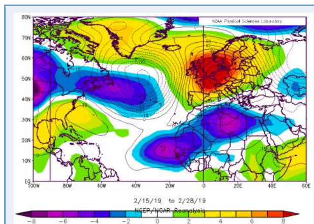
Figura 40 — Anomalías medias de geopotencial (contornos, mgp) y de temperatura en 850 hPa para el período 15-28 de febrero de 2019. Fuente NOAA/ESRL Physical Sciences Division.
