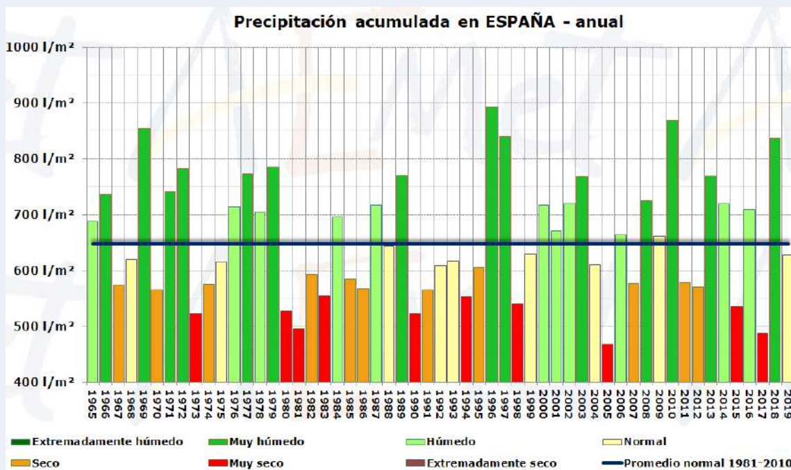
Figura 2 — Serie de precipitaciones medias anuales sobre España y carácter pluviométrico respecto al valor medio (período de referencia 1981-2010) desde 1965. Fuente AEMET.
