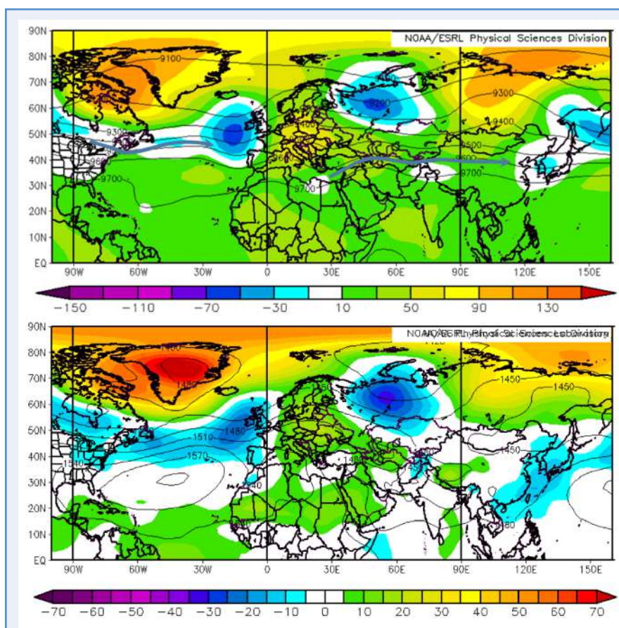
Figura 45 — Promedios de la altura del geopotencial y sus anomalías para los meses JJA; arriba: en 300 hPa (intervalo contorno 100 mgp); abajo en 850 hPa (intervalo contorno 30 mgp). Fuente NOAA/ESRL Physical Sciences Division.
