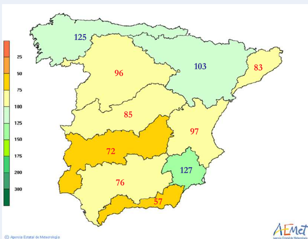
Figura 18 — Porcentaje de precipitación anual en 2019 sobre el valor normal (período de referencia 1981-2010) por grande cuencas o zonas características. Fuente AEMET.
