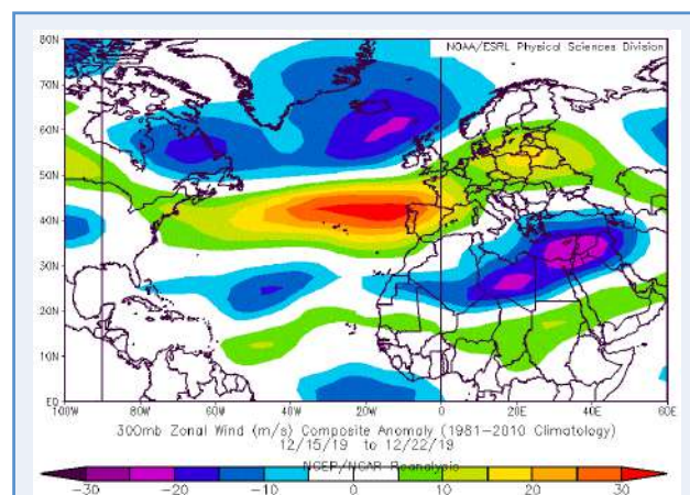
Figura 60 — Anomalías medias del viento zonal en 300 hPa para el período 15-22 de diciembre de 2019. Fuente NOAA/ESRL. ESRL Physical Sciences Division.
