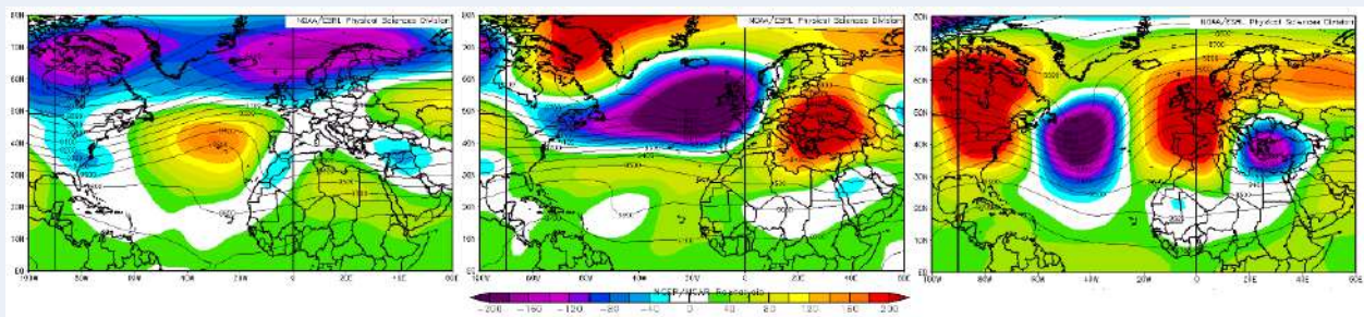
Figura 59 — Promedio de la altura del geopotencial (trazos finas) y sus anomalías (coloreadas) en 300 hPa para los días 1-14 (izquierda), 15-22 (centro), y 23-31 (derecha) de diciembre de 2019.
