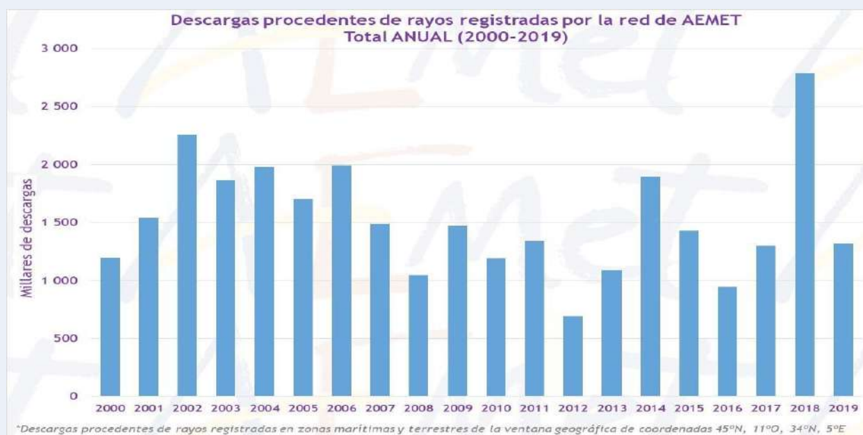
Figura 29 — Descargas totales anuales procedentes de rayos registradas por la red de AEMET (2000-2019). Fuente AEMET.
