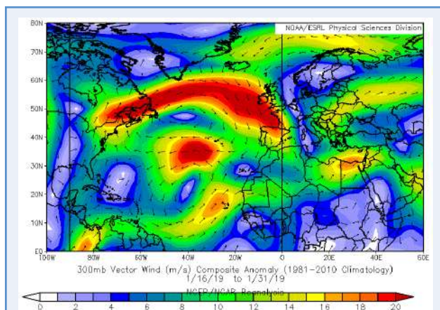
Figura 39 — Anomalías medias de viento en 300 hPa en el período 16 al 31 de enero. Fuente NOAA/ESRL Physical Sciences Division.
