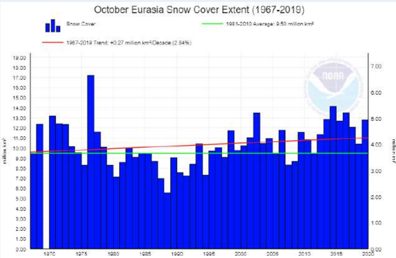
Figura 43 — Evolución histórica de la extensión de la cubierta de nieve euroasiática en octubre. (Fuente NOAA).
